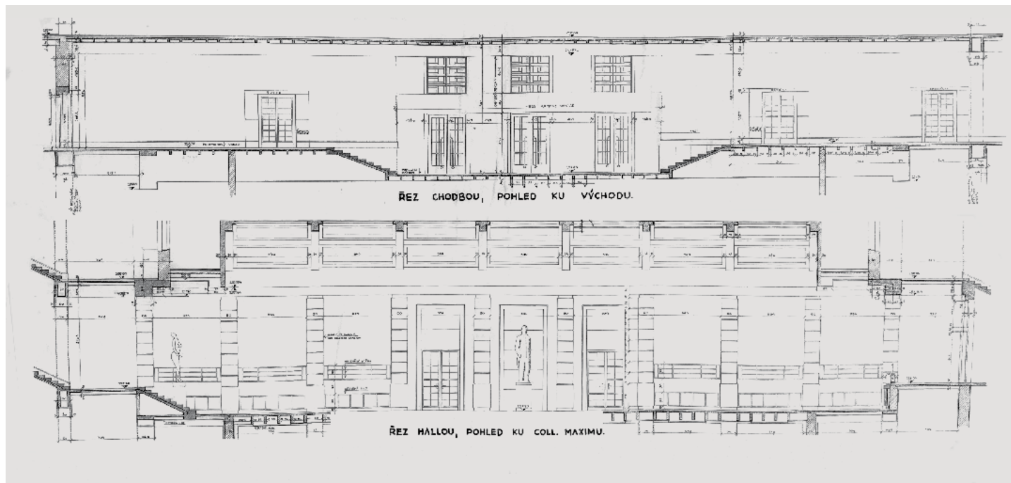
36 | Návrh architekta Aloise Dryáka, řez chodbou s pohledem na východ z budovy a řez vstupní halou s pohledem na vstup do Auditoria maxima (1929)
