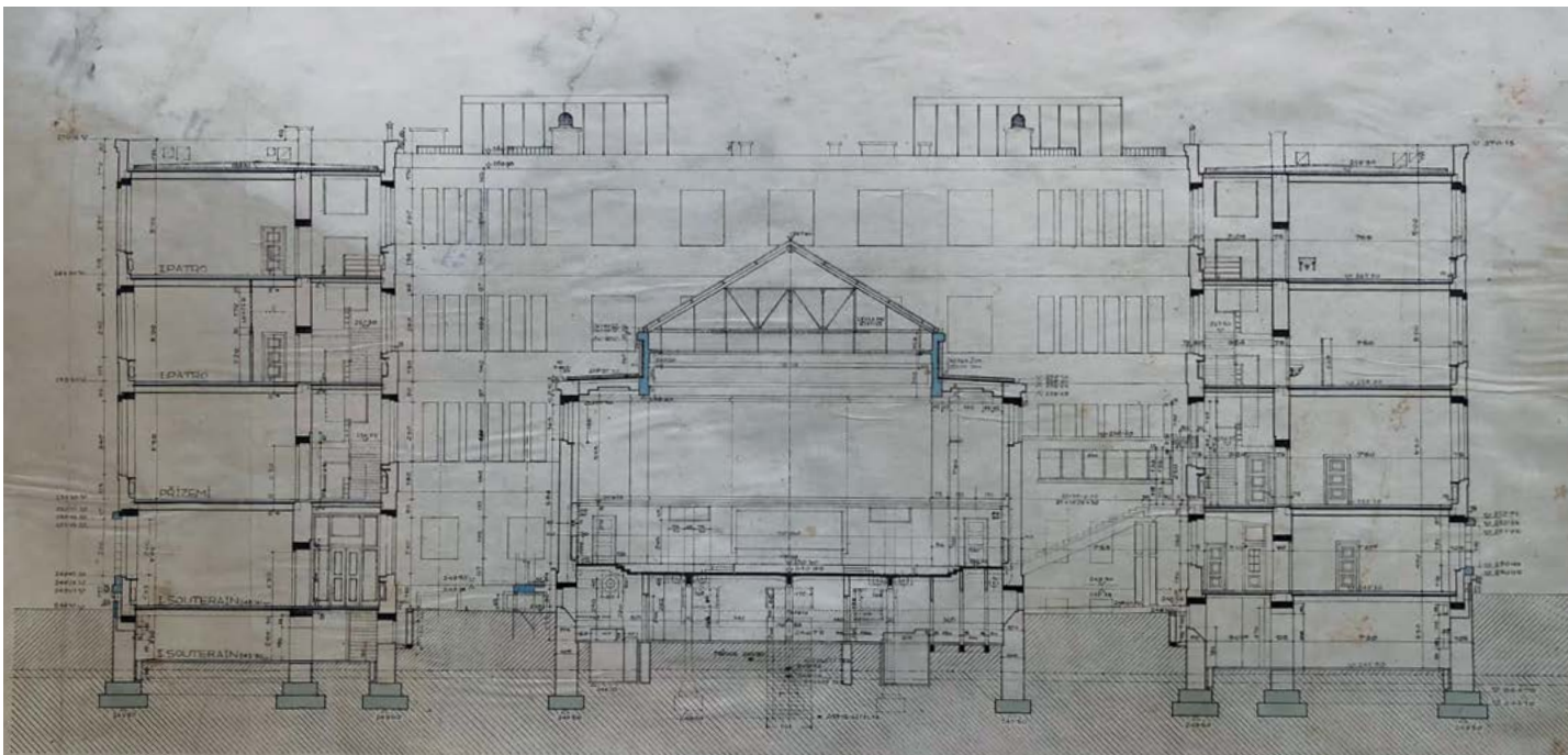
07 | Příčný řez budovou právnické fakulty
